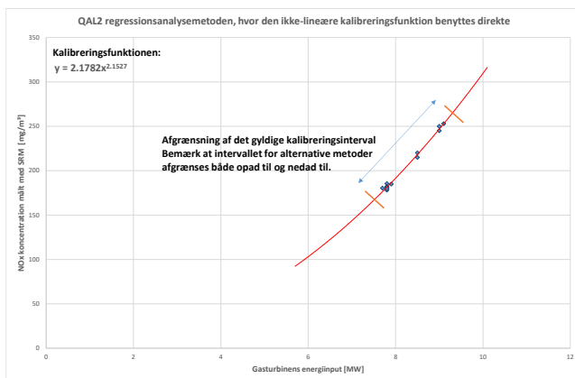
Figur 5 Eksempel på en ikke lineær QAL2 kalibreringsfunktion
