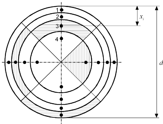
Figur 1 Illustration af den tangentielle metode til placering af målepunkter. Fra EN 13284-1.
