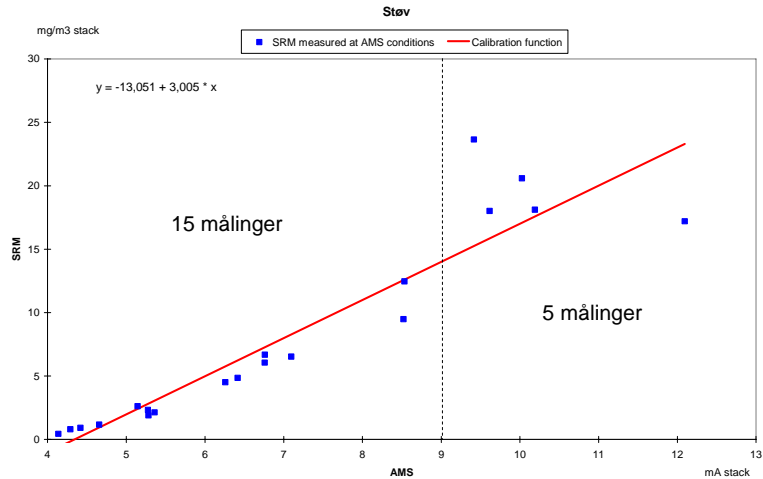
Figur 2-7 Eksempel på QAL2 målinger
